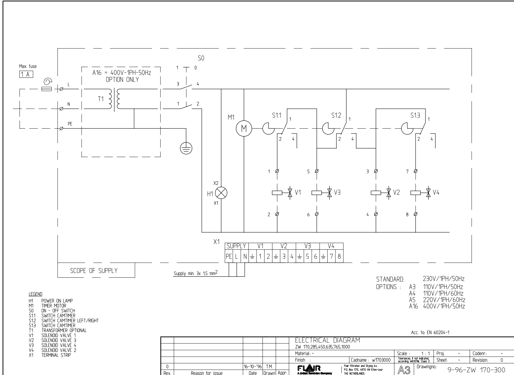
Esquema eléctrico, versiones CA
