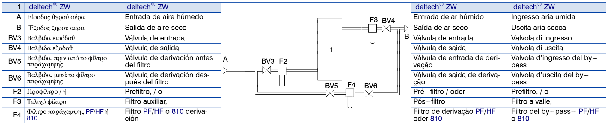
Fig. 2 Διάταξη ηηλώματος πεπιεσμένου αέρα
